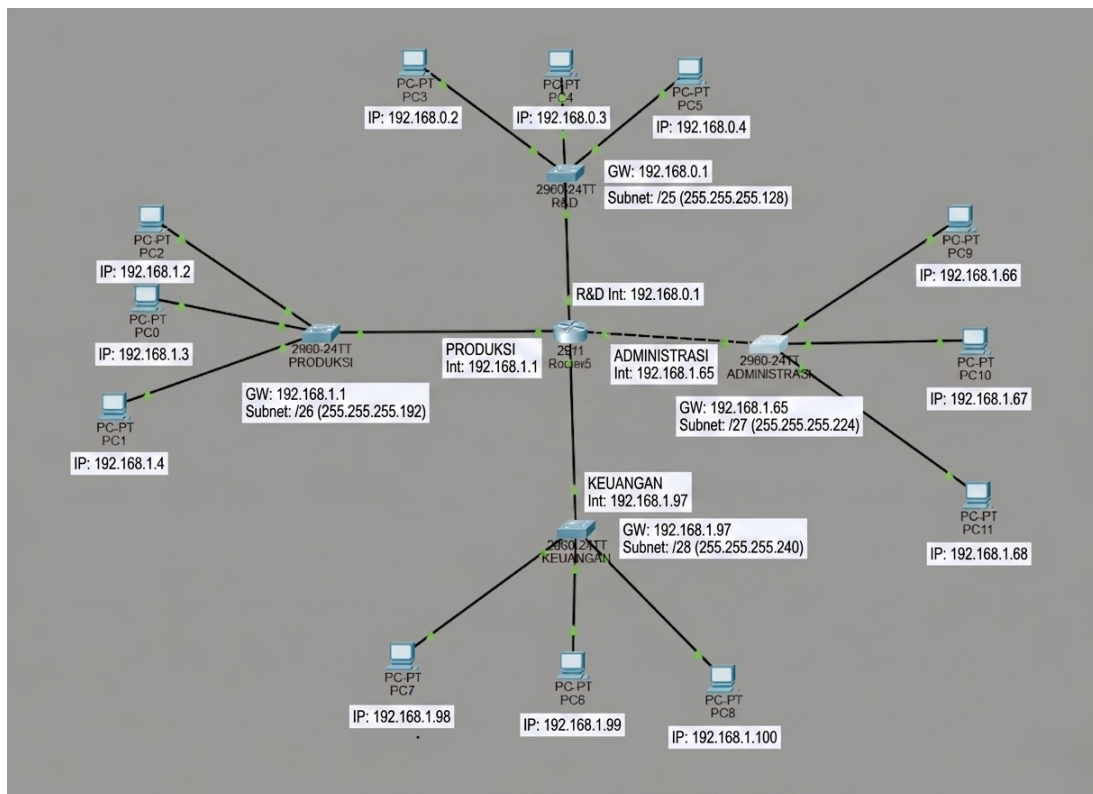
Gambar 1: Topologi Jaringan Perusahaan
